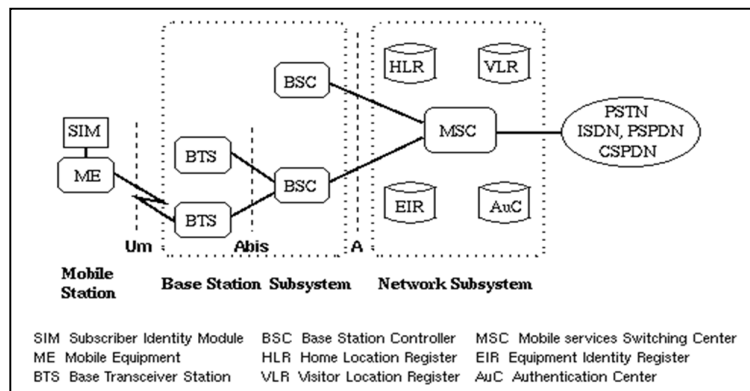
GAMBAR 3. Struktur Jaringan GSM.
