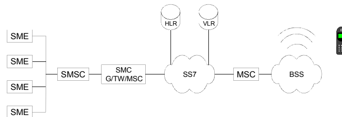
GAMBAR 4. Arsitektur Jaringan SMS.
