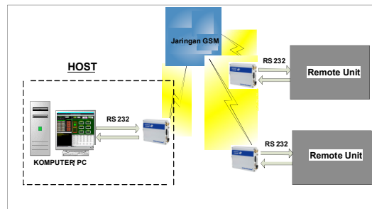
GAMBAR 5. Diagram Blok Host Mini SCADA.
